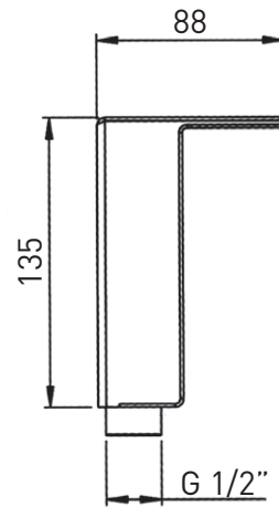
6105 CASSIOPEA - INOX - SOFFIONI E BRACCI
