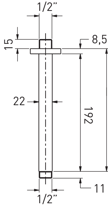
3720 - OTTONE - SOFFIONI E BRACCI
